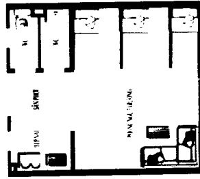
MẶT BẰNG PHÒNG Ớ MẪU NHÀ 2.1
